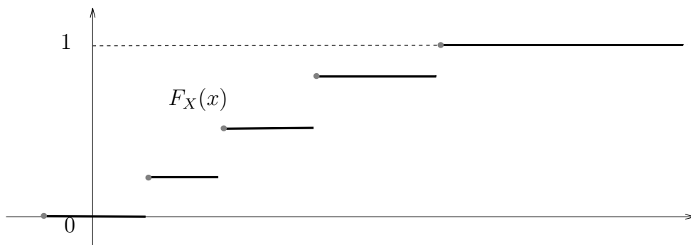
FIGURE 3.3 – Fonction de répartition d'une variable discrète.
