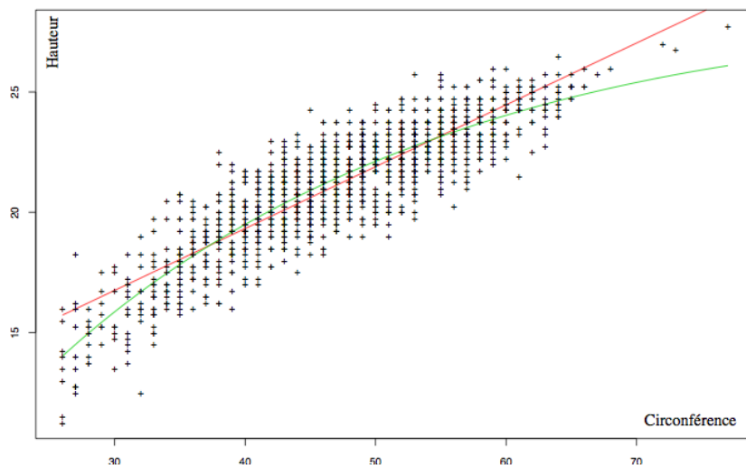
FIGURE 7.4 – En rouge la régression linéaire du type Y = aX + b du nuage de points. En vert, la régression de type Y = aX + b\sqrt{X} + c qui semble mieux adaptée aux données.
