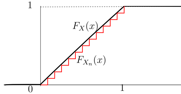
FIGURE 4.1 – Fonction de répartition des lois uniformes continue et discrètes.
