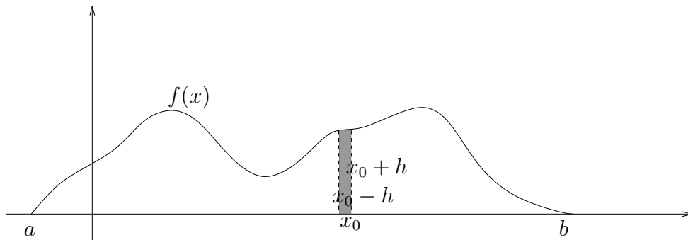
FIGURE 3.1 – Probabilité sur un intervalle via une densité.
