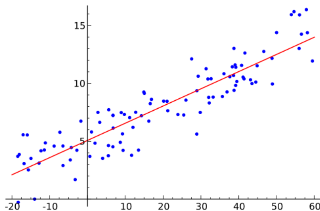
FIGURE 7.1 – Nuage de points et droite de régression.
