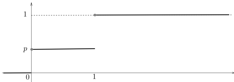
FIGURE 3.4 – Fonction de répartition d'une variable de Bernoulli \mathcal{B}(p) .
