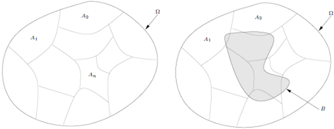
FIGURE 2.1 – Probabilité conditionnelle et partition.
