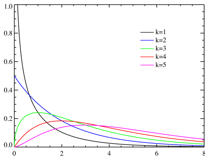
FIGURE 6.1 – Allure des densités des lois \chi^2(k) pour différentes valeurs de k .
