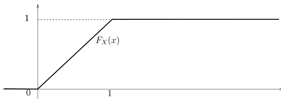
FIGURE 3.7 – Fonction de répartition d'une variable uniforme.
