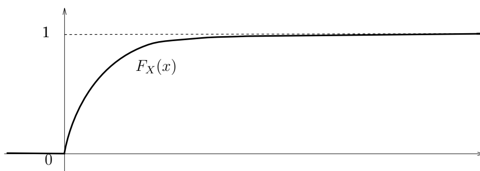
FIGURE 3.8 – Fonction de répartition d'une variable exponentielle.
