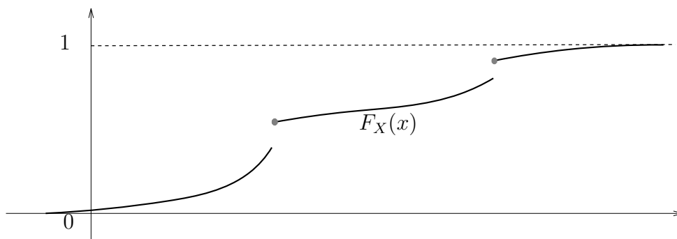
FIGURE 3.2 – Fonction de répartition générique.
