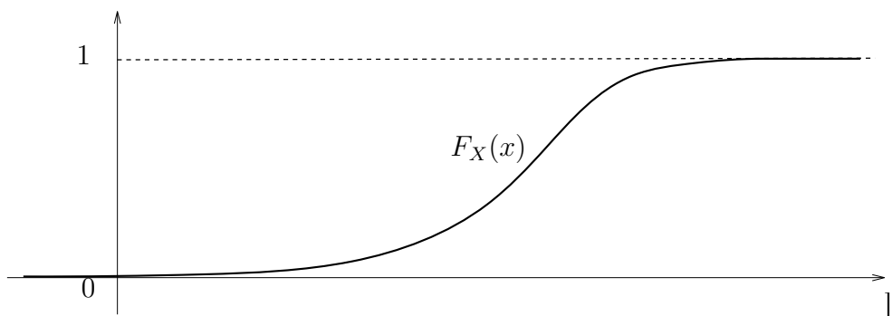
FIGURE 3.6 – Fonction de répartition d'une variable continue.
