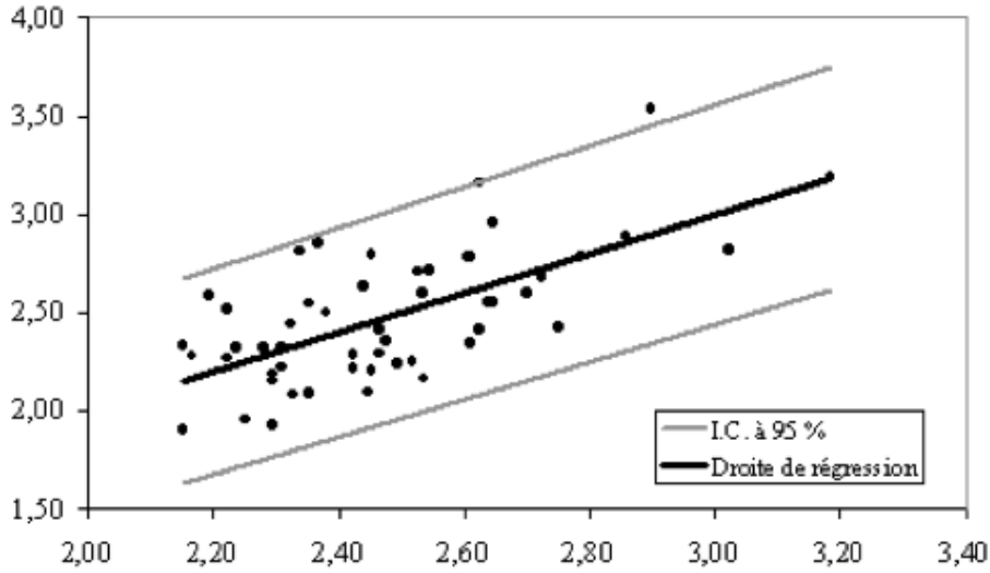
FIGURE 7.2 – Exemple d'intervalle de confiance pour la prédiction.
