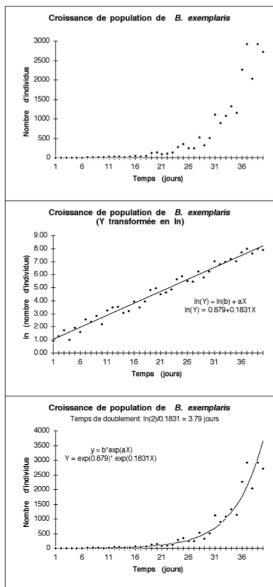
FIGURE 7.3 – Modèle exponentiel Y = be^{aX} et regression linéaire.
