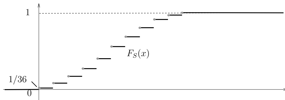
FIGURE 3.5 – Fonction de répartition de la variable S (somme de deux dés).
