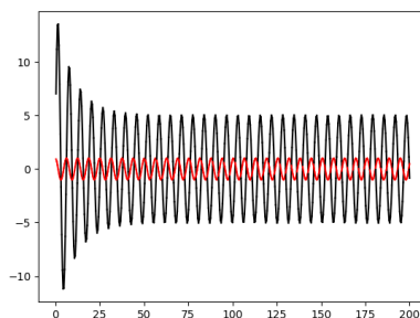
f'' + f'/5 + f = \cos(t) : résonance, \omega = \omega_0 = 1 en rouge l'excitation et en noir la réponse de l'oscillateur
