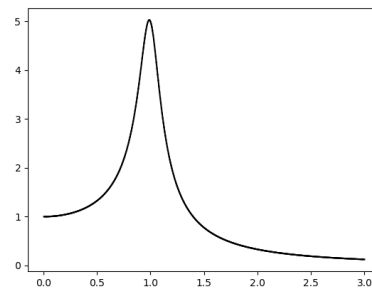
amplitude lorsque f'' + f'/5 + f = \cos(\omega t)
