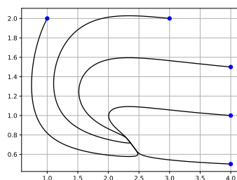
système de Holling et MacArthur-Rosenzweig K = 3, c = 0.7, e = 1
