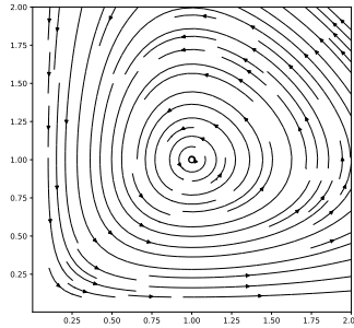
système de Lotka-Volterra lorsque a = b = c = d = 1
