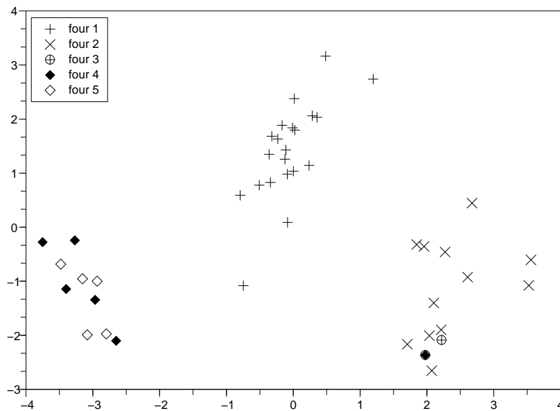
Répartition des poteries selon les 5 fours dans les deux premières composantes principales normalisées
