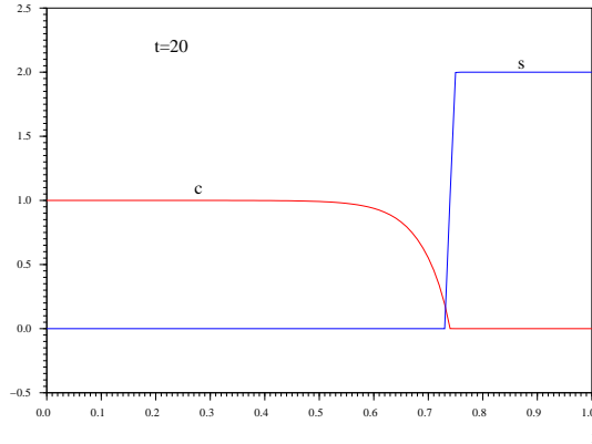
FIG. 2. c et s en fonction de x à t = 20 , avec k = 10^4 .
