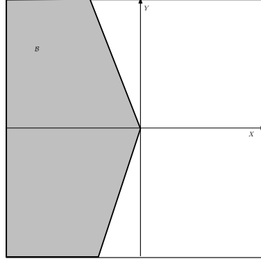
Fig. 2.1. Cone \mathcal{B}
